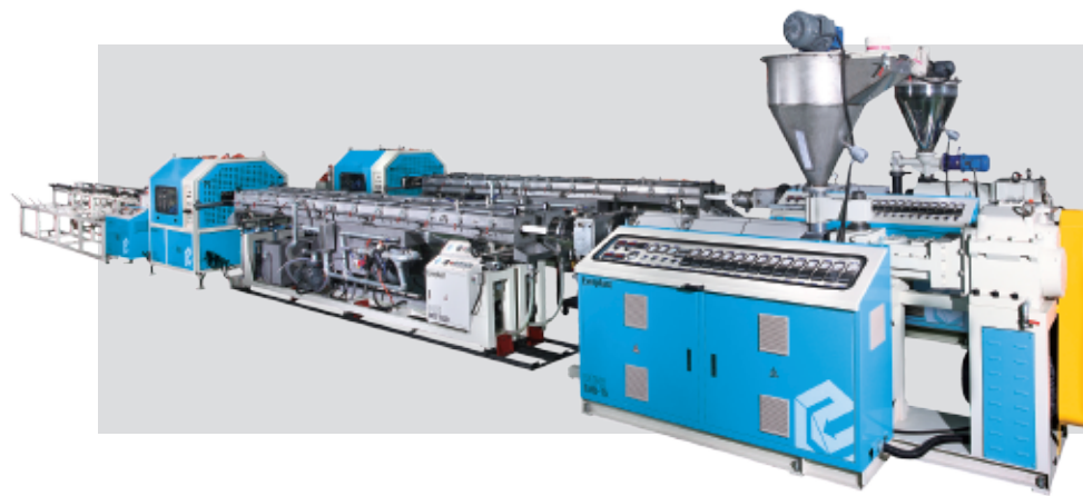
PVC 管(雙出)
